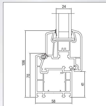
Profilschnitt
