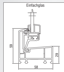
Einfachglas
